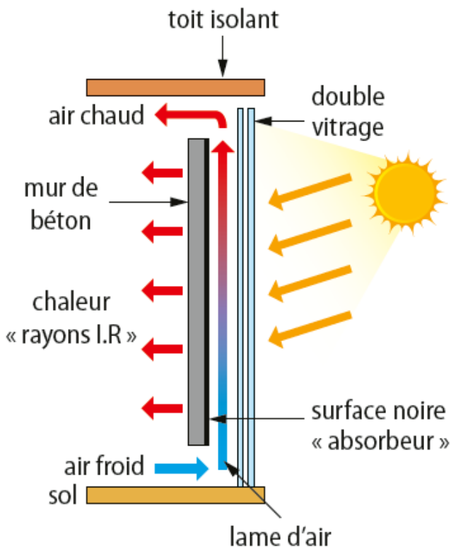
Schéma fonctionnel d'un mur trombe
